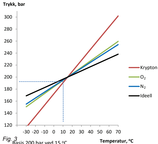
Sammenheng mellom temperatur og trykk for permanente gasser
