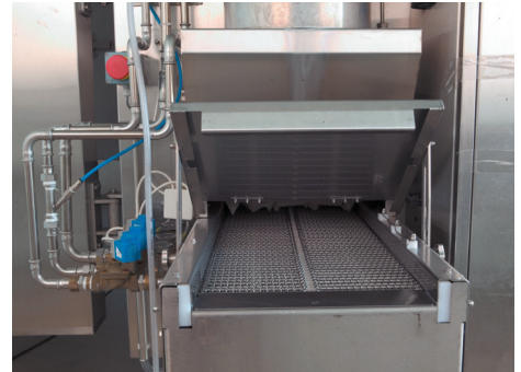
Innmating. Rørapplegg med tilhørende ventiler for rengjøring vises på siden
